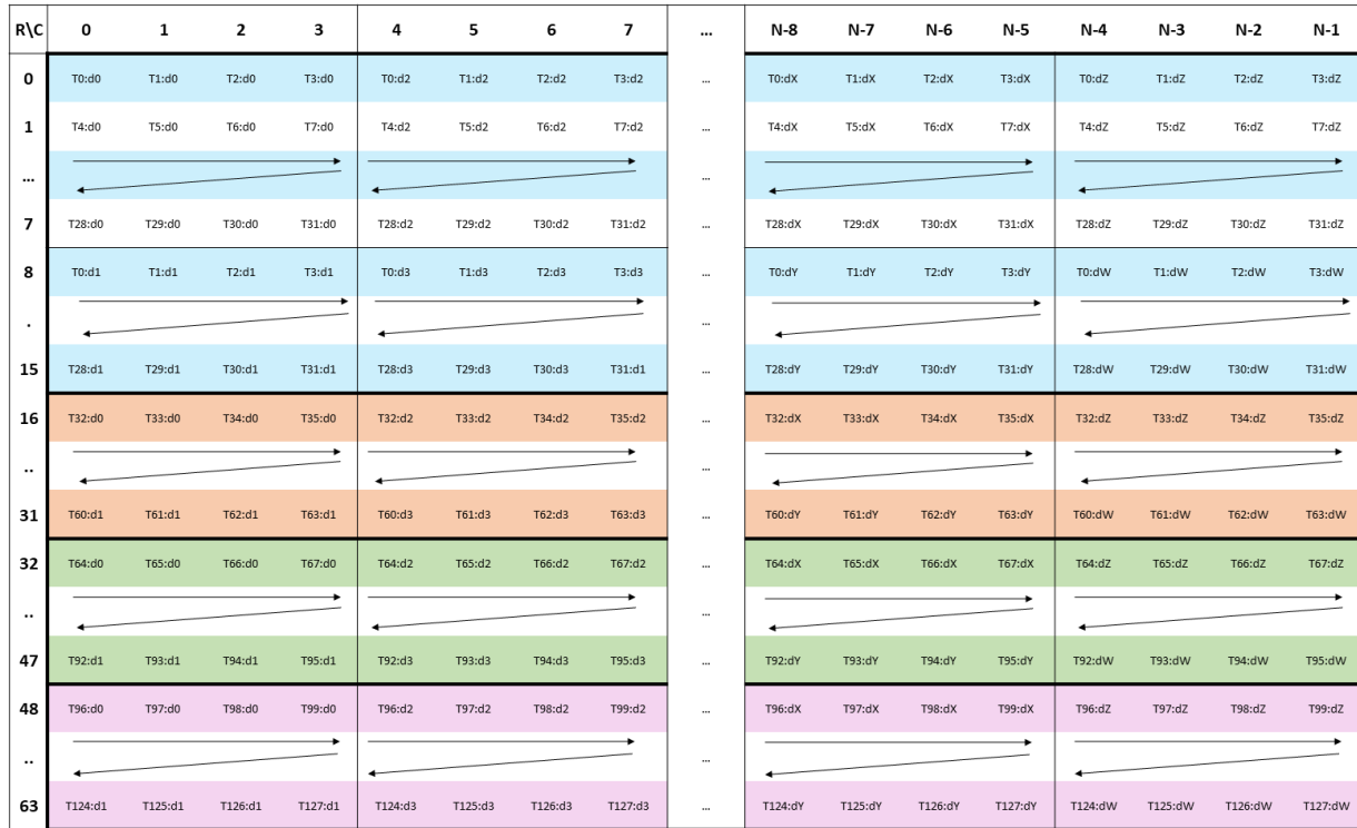
(tid % 128) : fragments
