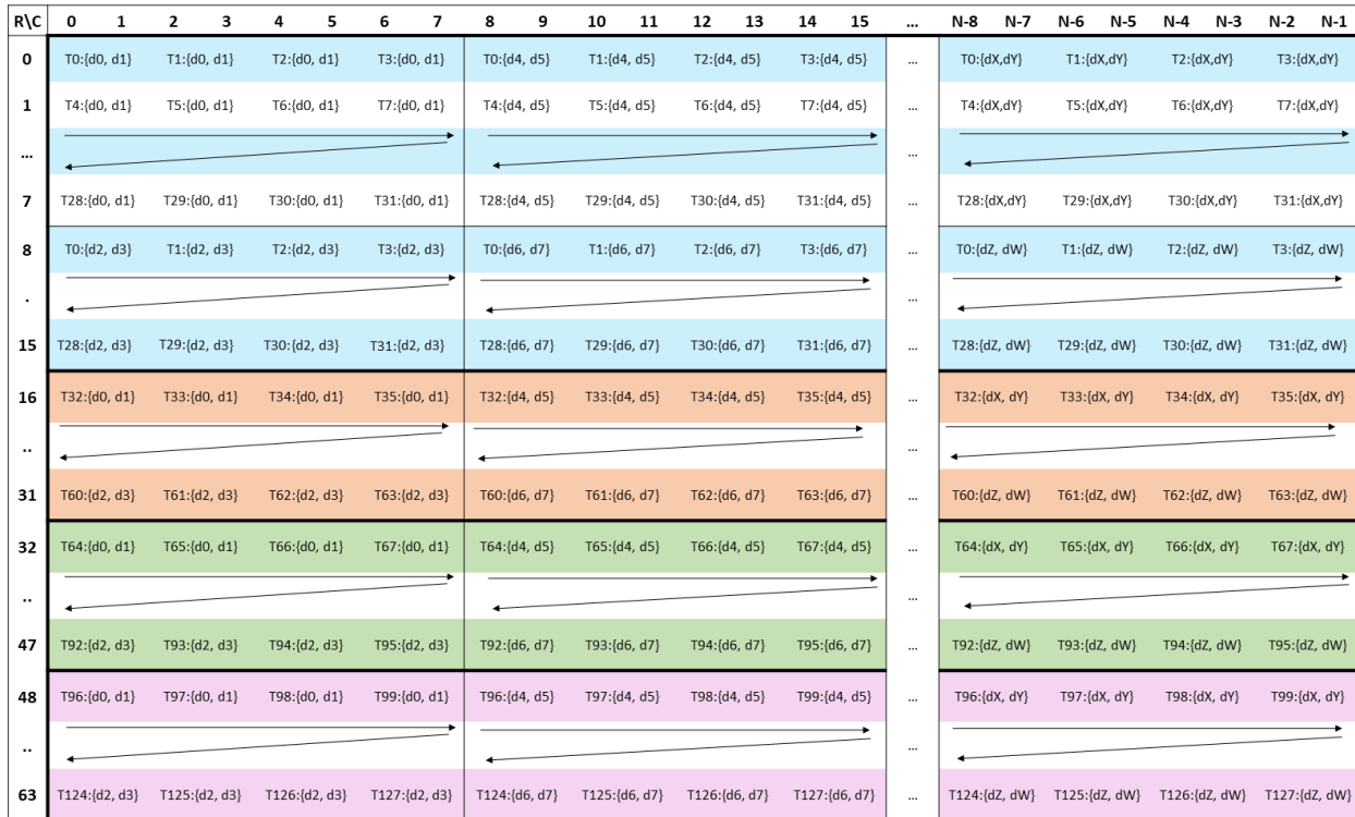
(tid % 128) : fragments
